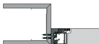
Tirare | Parete Cartongesso 125 mm
