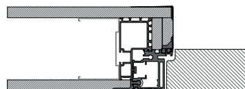
Tirare | Parete Cartongesso 100 mm
