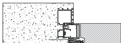
Spingere | Parete Muratura 100 mm
