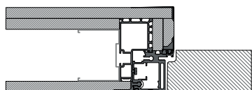
Tirare | Parete Cartongesso 100 mm
