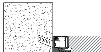
Spingere | Parete Muratura 150 mm
