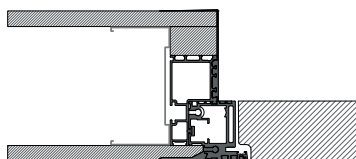
Spingere | Parete Cartongesso 125 mm
