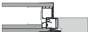
Spingere | Parete Cartongesso 100 mm
