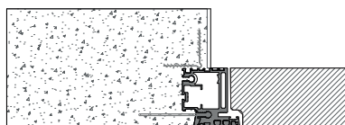
Spingere | Parete Muratura 100 mm
