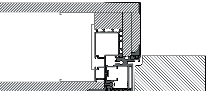
Tirare | Parete Cartongesso 125 mm
