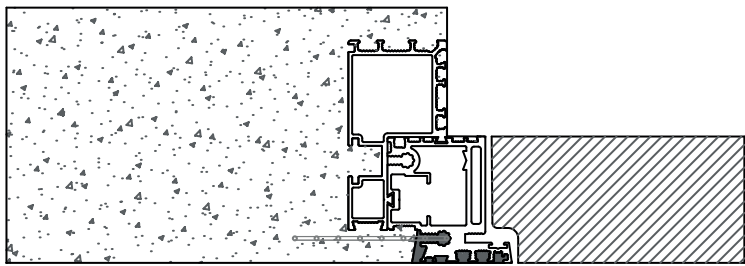
Spingere | Parete Muratura 100 mm
