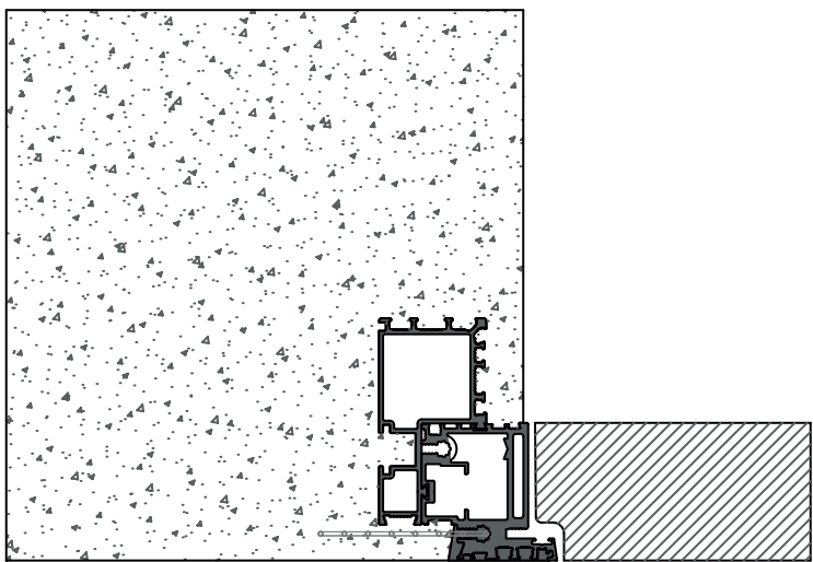
Spingere | Parete Muratura 200 mm
