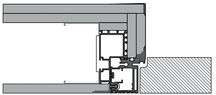
Tirare | Parete Cartongesso 125 mm
