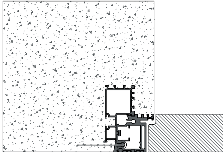
Tirare | Parete Muratura 200 mm
