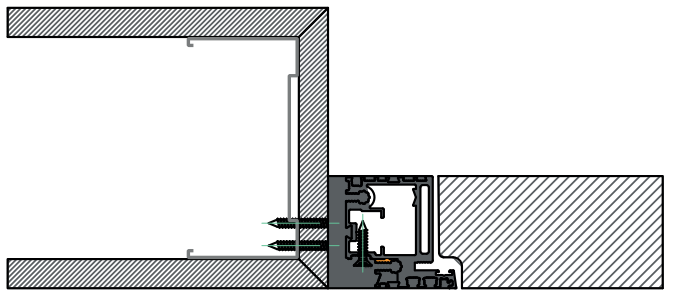
Spingere | Parete Cartongesso 125 mm
