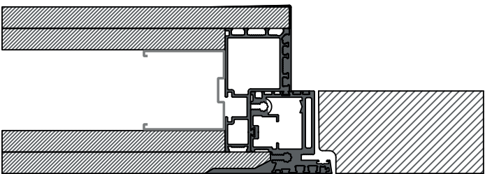
Spingere | Parete Cartongesso 100 mm
