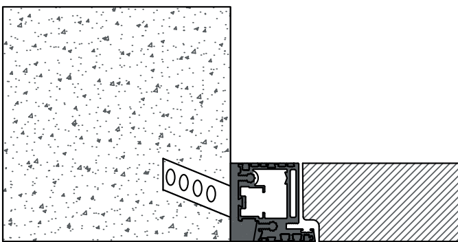
Spingere | Parete Muratura 150 mm
