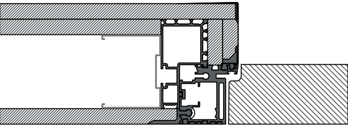
Tirare | Parete Cartongesso 100 mm
