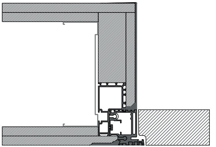
Spingere | Parete Cartongesso 200 mm
