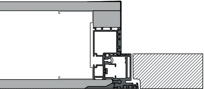
Spingere | Parete Cartongesso 125 mm
