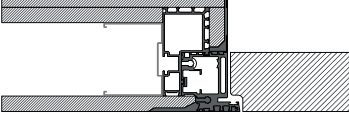
Spingere | Parete Cartongesso 100 mm
