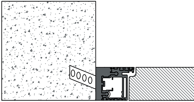
Tirare | Parete Muratura 150 mm
