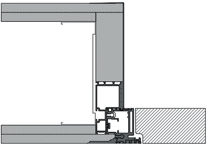
Spingere | Parete Cartongesso 200 mm
