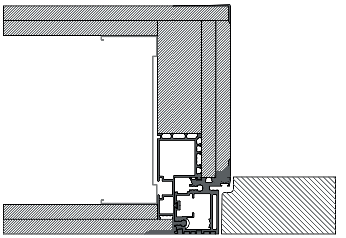
Tirare | Parete Cartongesso 200 mm
